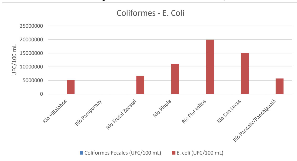
Gráfica 11: Valores de Coliformes fecales y Escherichia coli (UFC/100 ml) detectados en los ríos monitoreados en la Cuenca del Lago de Amatitlán durante el mes de noviembre, 2024.
