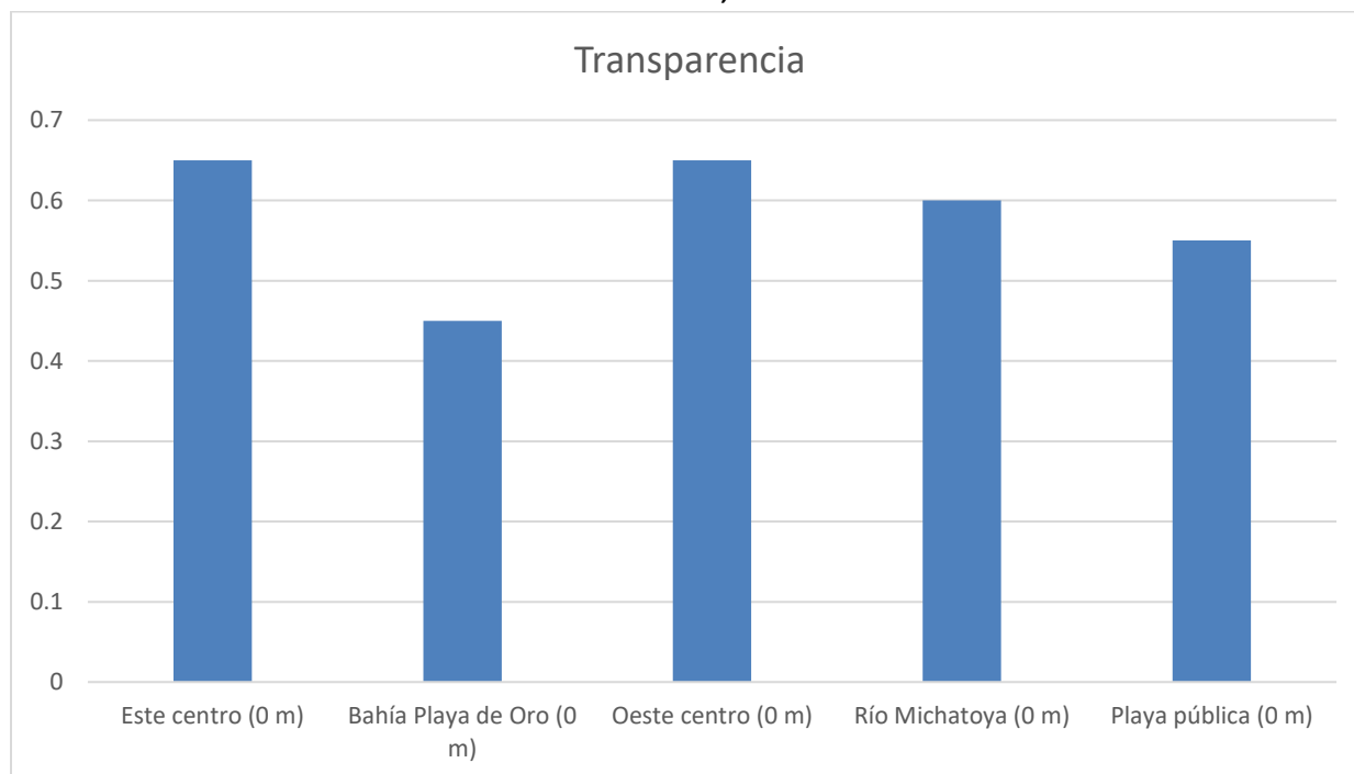
Gráfica 12: Transparencia (m) registrada en cinco puntos de monitoreo del lago de Amatitlán durante el mes de noviembre, 2024
