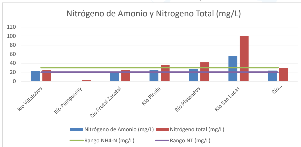
Gráfica 6: Valores de nitrógeno total (N) y amonio ( \text{NH}_3\text{-N} ) de los ríos monitoreados en la Cuenca del Lago de Amatitlán durante el mes de noviembre, 2024.
