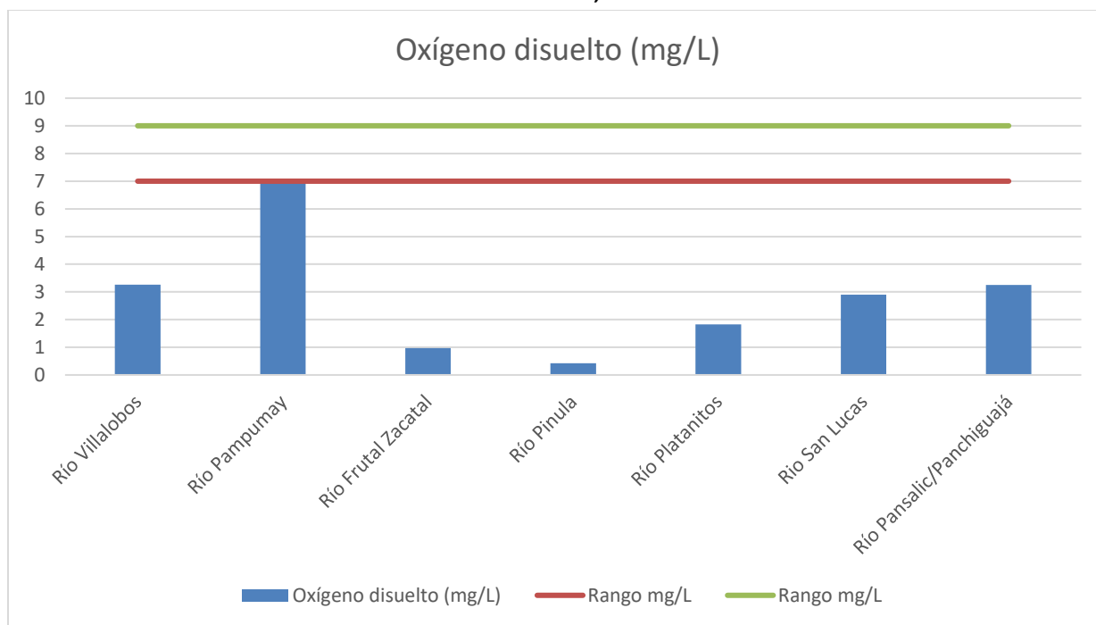
Gráfica 4: Oxígeno disuelto (mg/L) de los ríos monitoreados en la Cuenca del Lago de Amatitlán durante el mes de noviembre, 2024.
