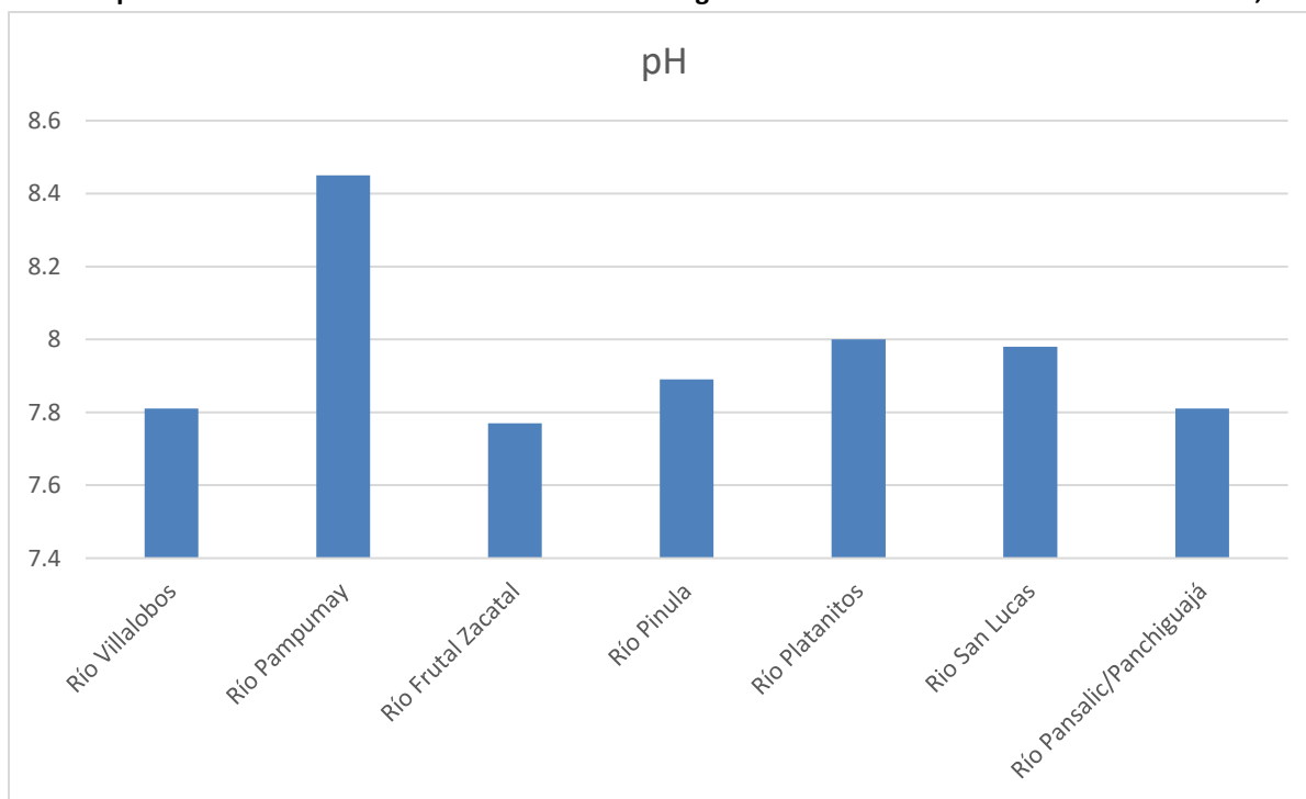
Gráfica 1: pH de los ríos monitoreados en la Cuenca del Lago de Amatitlán durante el mes de noviembre, 2024.
