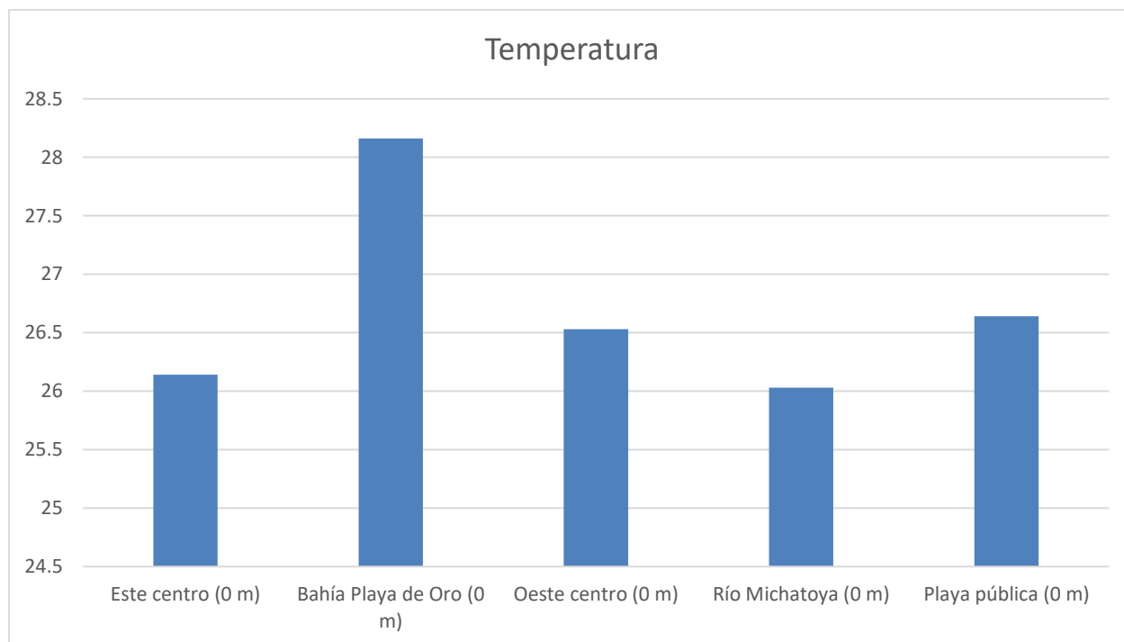
Gráfica 14: Perfil de temperatura (°C) en los puntos de monitoreo que tienen profundidad en el lago de Amatitlán (Este y Oeste Centro), durante el mes de noviembre, 2024.
