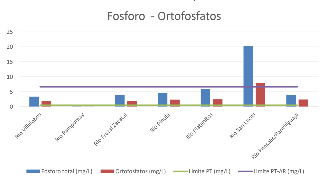
Gráfica 8: Valores de fósforo total (P) y ortofosfatos (PO4-P) de los ríos monitoreados en la Cuenca del Lago de Amatitlán durante el mes de noviembre, 2024.
