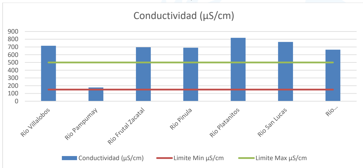
Gráfica 3: Conductividad ( \mu\text{S}/\text{cm} ) de los ríos monitoreados en la Cuenca del Lago de Amatitlán durante el mes de noviembre, 2024.
