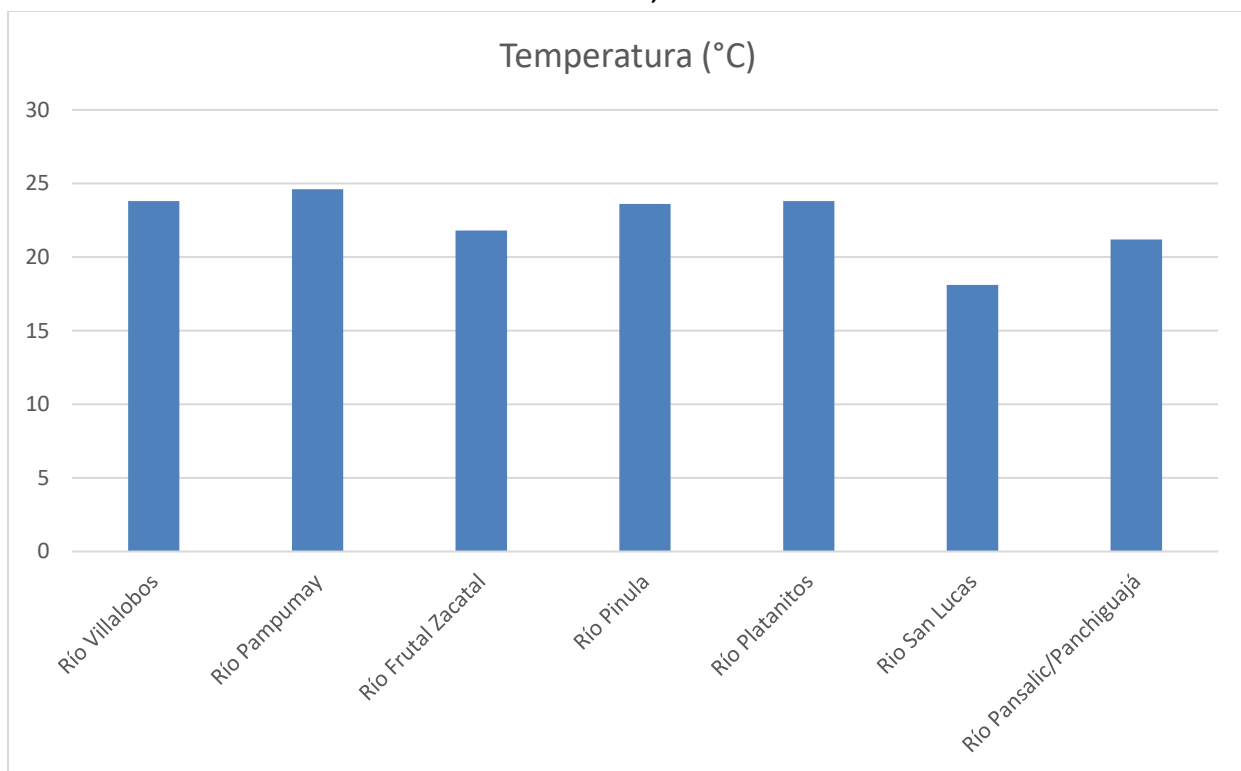
Gráfica 2: Temperatura (°C) de los ríos monitoreados en la Cuenca del Lago de Amatitlán durante el mes de noviembre, 2024.
