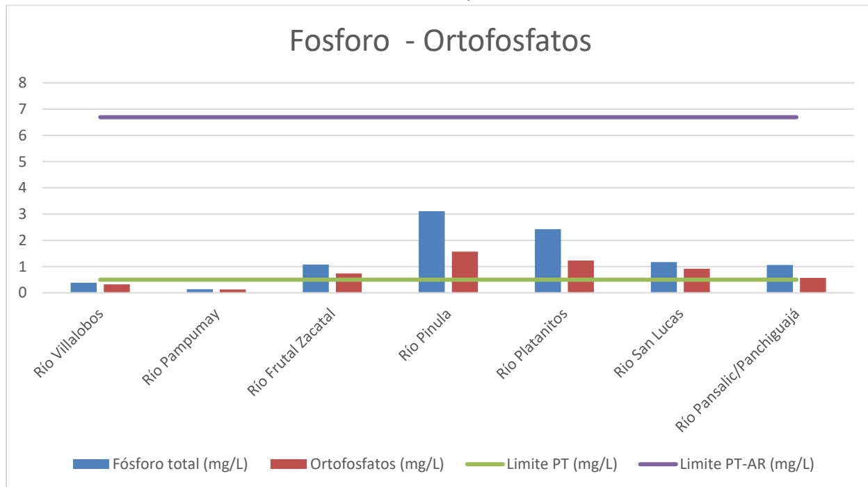
Gráfica 8: Valores de fósforo total (P) y ortofosfatos (PO4-P) de los ríos monitoreados en la Cuenca del Lago de Amatitlán durante el mes de julio, 2024.
