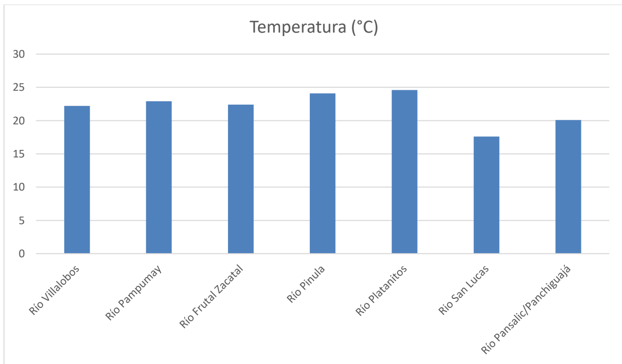
Gráfica 2: Temperatura (°C) de los ríos monitoreados en la Cuenca del Lago de Amatitlán durante el mes de julio, 2024.
