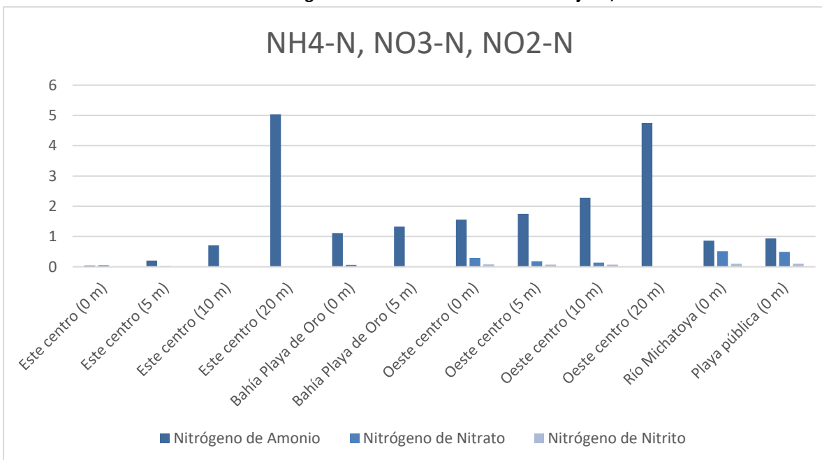
Gráfica 17: Valores de amonio ( \text{NH}_4\text{-N} ), nitratos ( \text{NO}_3\text{-N} ) y nitritos ( \text{NO}_2\text{-N} ) detectados en cinco puntos de monitoreo del lago de Amatitlán durante el mes de julio, 2024.
