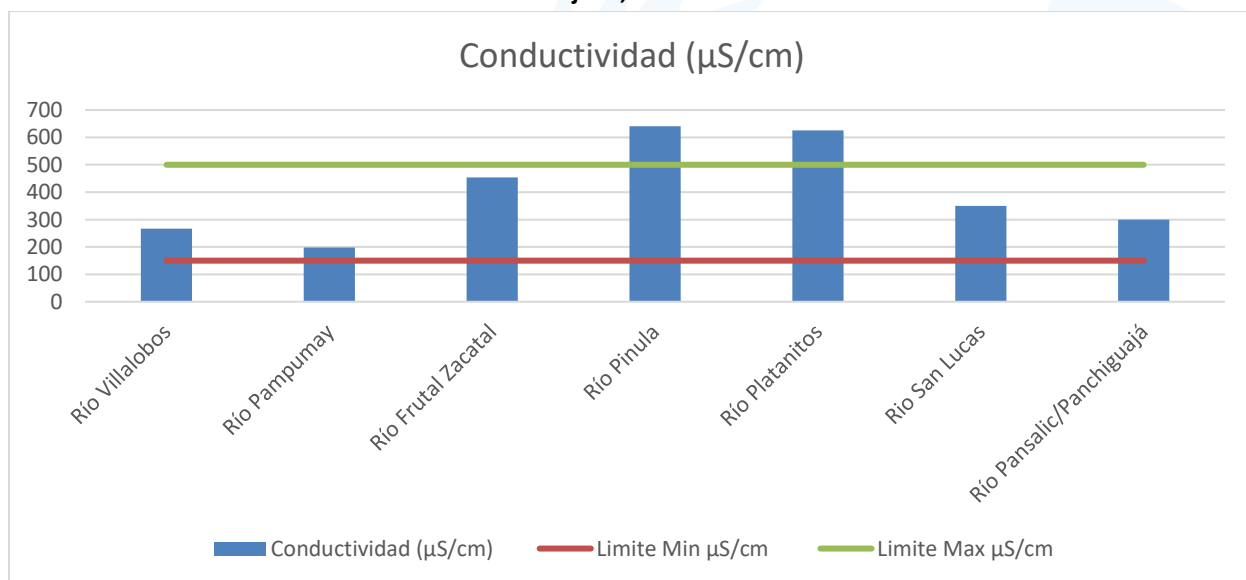
Gráfica 3: Conductividad ( \mu\text{S}/\text{cm} ) de los ríos monitoreados en la Cuenca del Lago de Amatitlán durante el mes de julio, 2024.
