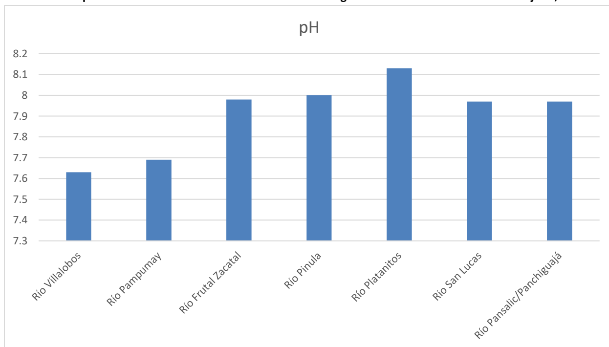
Gráfica 1: pH de los ríos monitoreados en la Cuenca del Lago de Amatitlán durante el mes de julio, 2024.
