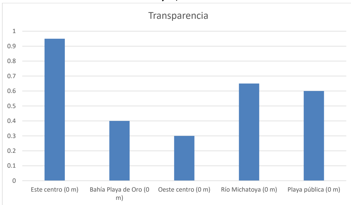
Gráfica 12: Transparencia (m) registrada en cinco puntos de monitoreo del lago de Amatitlán durante el mes de julio, 2024
