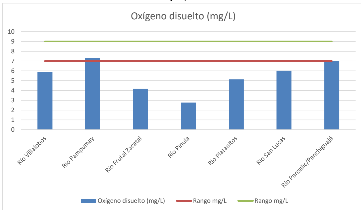
Gráfica 4: Oxígeno disuelto (mg/L) de los ríos monitoreados en la Cuenca del Lago de Amatitlán durante el mes de julio, 2024.
