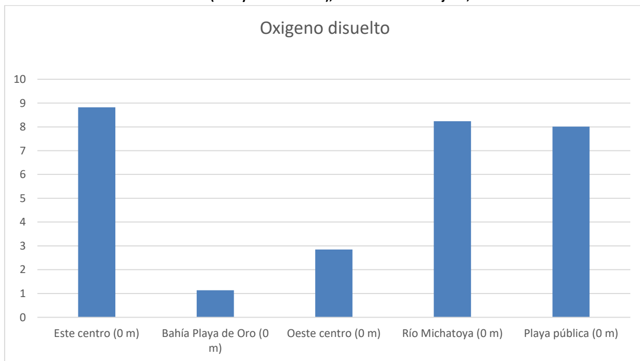
Gráfica 13: Perfil de oxígeno disuelto (mg/L) en los puntos de monitoreo que tienen la profundidad en el lago de Amatitlán (Este y Oeste Centro), durante el mes de julio, 2024
