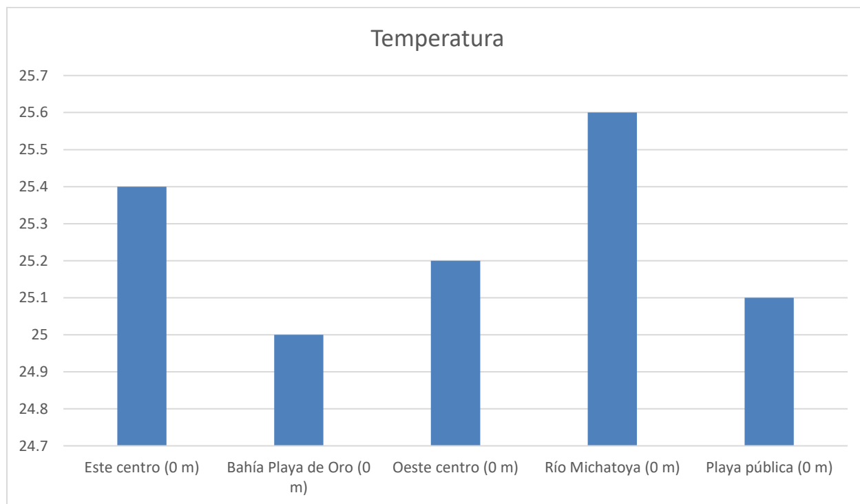
Gráfica 14: Perfil de temperatura (°C) en los puntos de monitoreo que tienen profundidad en el lago de Amatitlán (Este y Oeste Centro), durante el mes de julio, 2024.
