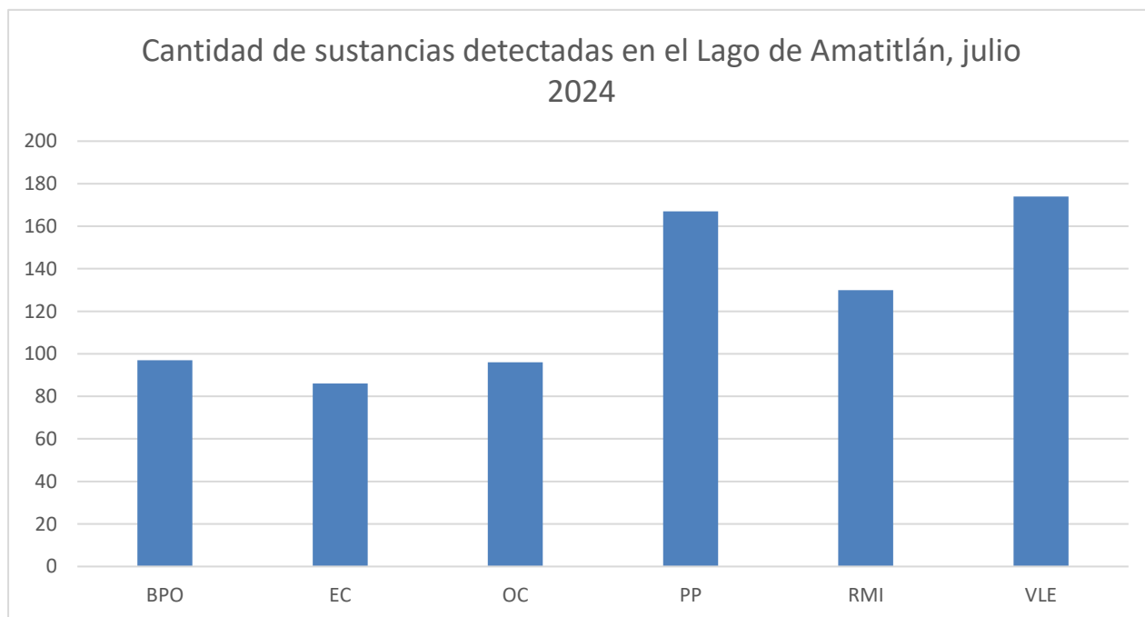
Gráfica 18: Cantidad de Sustancias Orgánicas detectadas en seis puntos de monitoreo del lago de Amatitlán durante el mes de marzo y abril, 2024.
