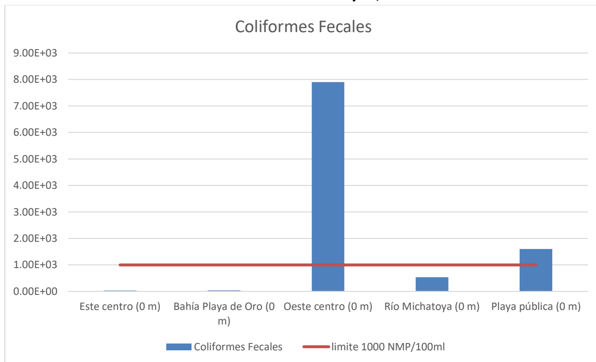
Gráfica 19: Valores de coliformes fecales (UFC/100 ml) registrados en cinco puntos de monitoreo del lago de Amatitlán durante el mes de julio, 2024.
