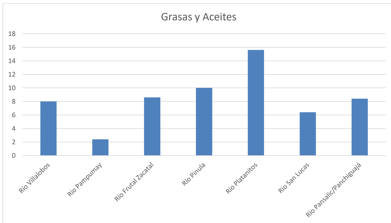
Gráfica 10: Valores de grasas y aceites (mg/L) en los ríos monitoreados de la cuenca del lago de Amatitlán durante el mes de julio, 2024.
