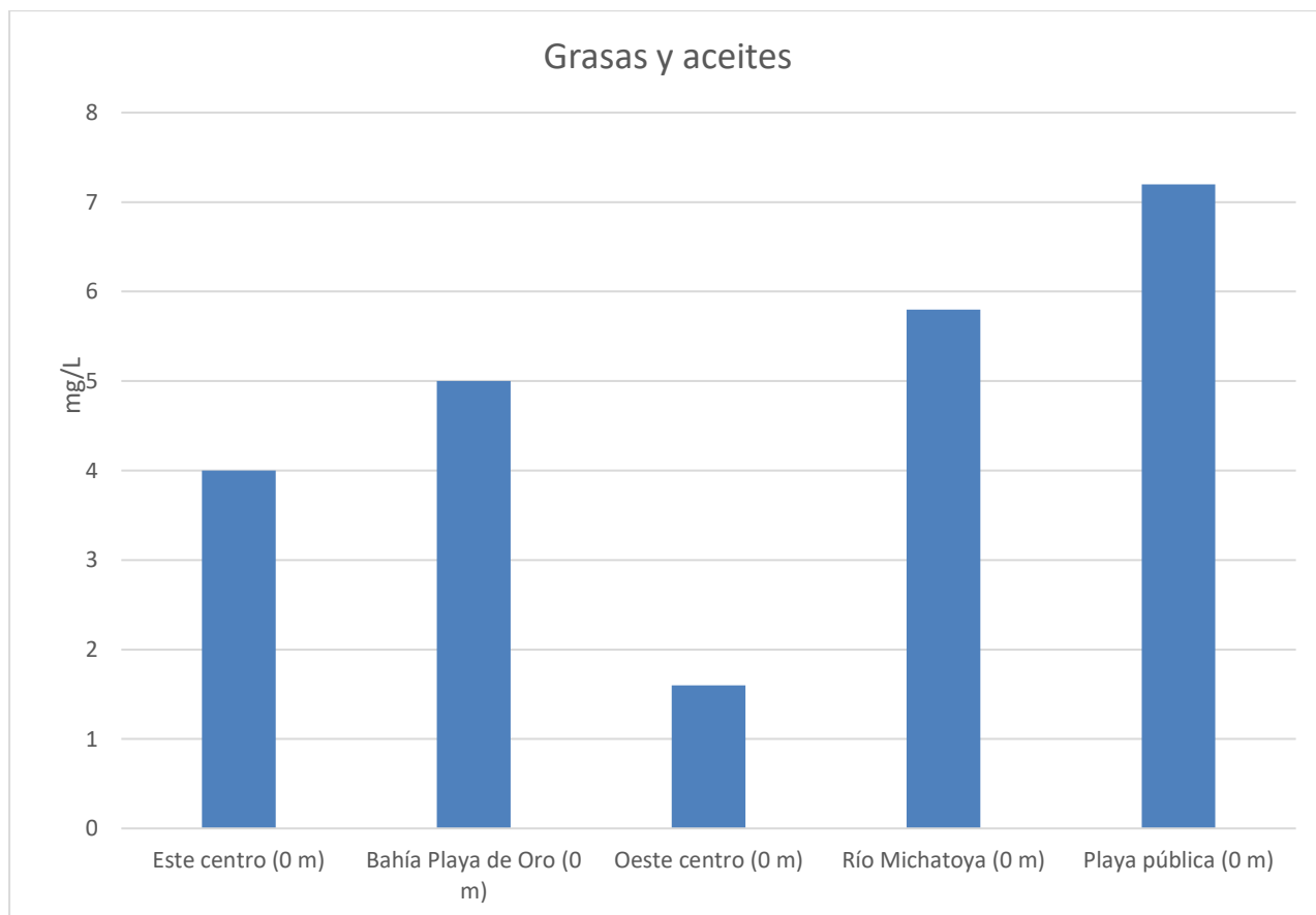
Gráfica 18: Valores de grasas y aceites (mg/L) registrados en cinco puntos de monitoreo del lago de Amatitlán durante el mes de julio, 2024.
