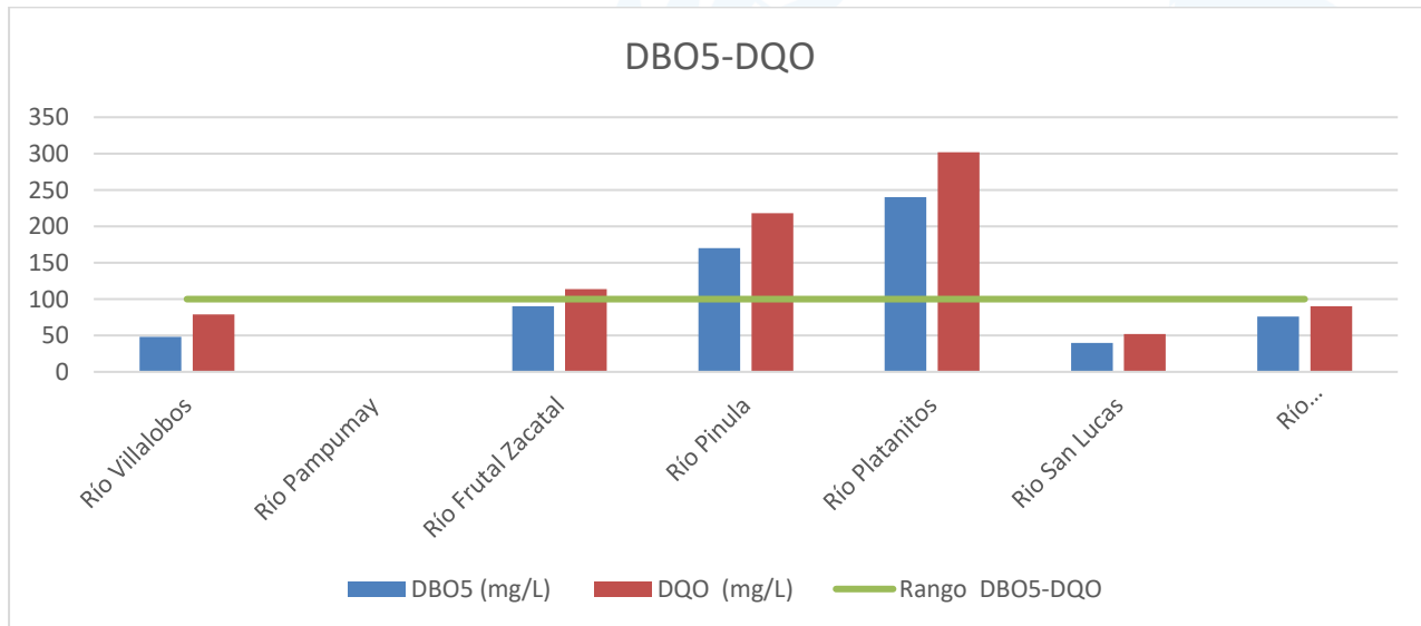
Gráfica 9: Valores de DBO 5 y DQO de los ríos muestreados de la Cuenca del lago de Amatitlán durante el mes de julio, 2024.
