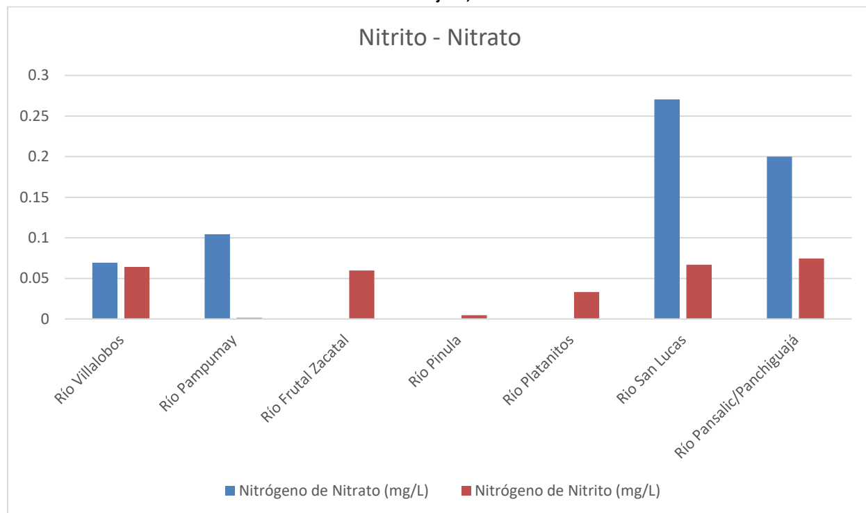
Gráfica 7: Valores de nitratos (NO 3 -N) y nitritos (NO 2 -N) de los ríos monitoreados en la Cuenca del Lago de Amatitlán durante el mes de julio, 2024.
