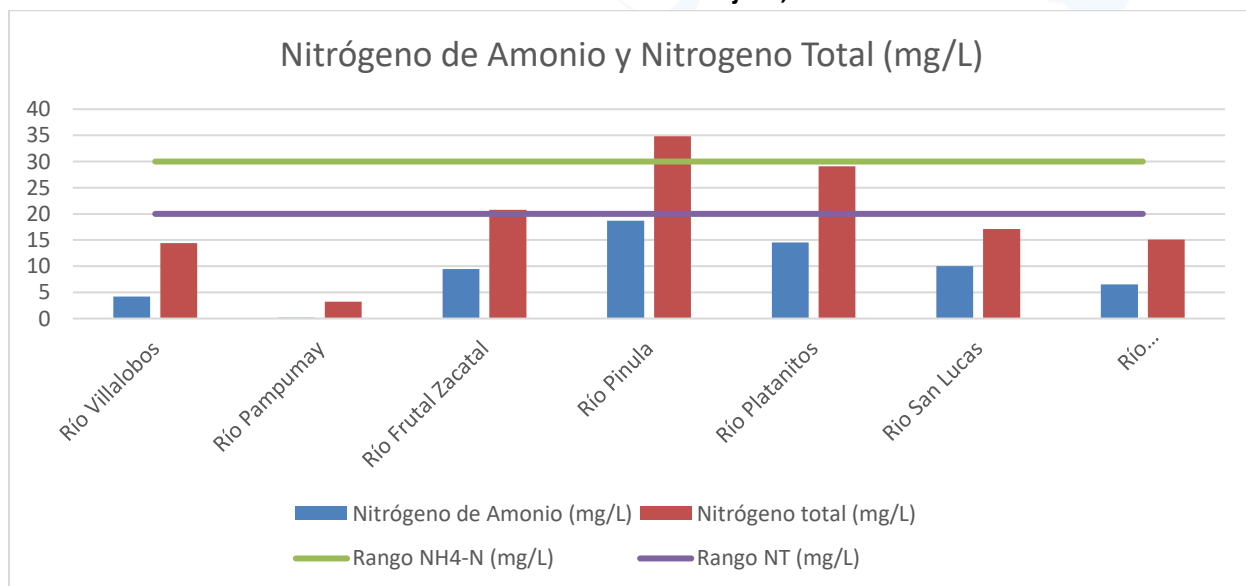
Gráfica 6: Valores de nitrógeno total (N) y amonio ( \text{NH}_3\text{-N} ) de los ríos monitoreados en la Cuenca del Lago de Amatitlán durante el mes de julio, 2024.
