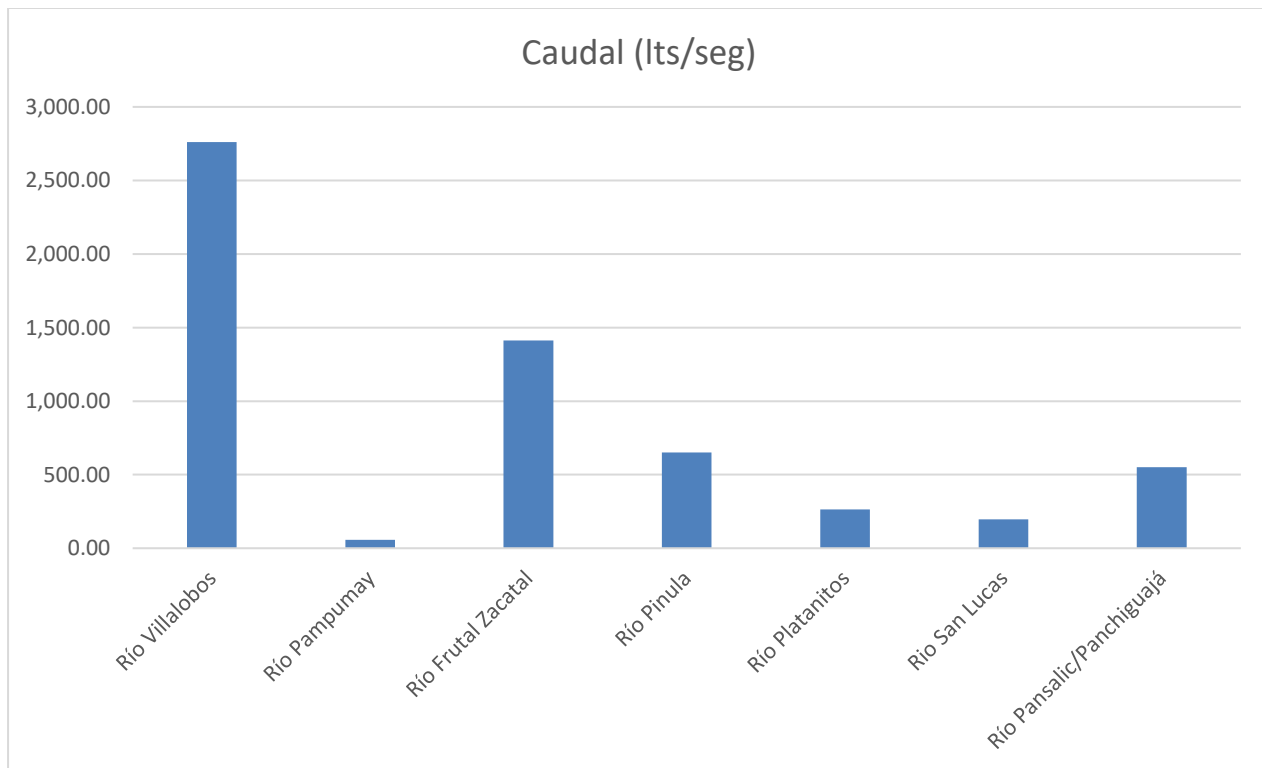
Gráfica 5: Caudal (lt/s) de los ríos monitoreados en la Cuenca del Lago de Amatitlán durante el mes de julio, 2024.
