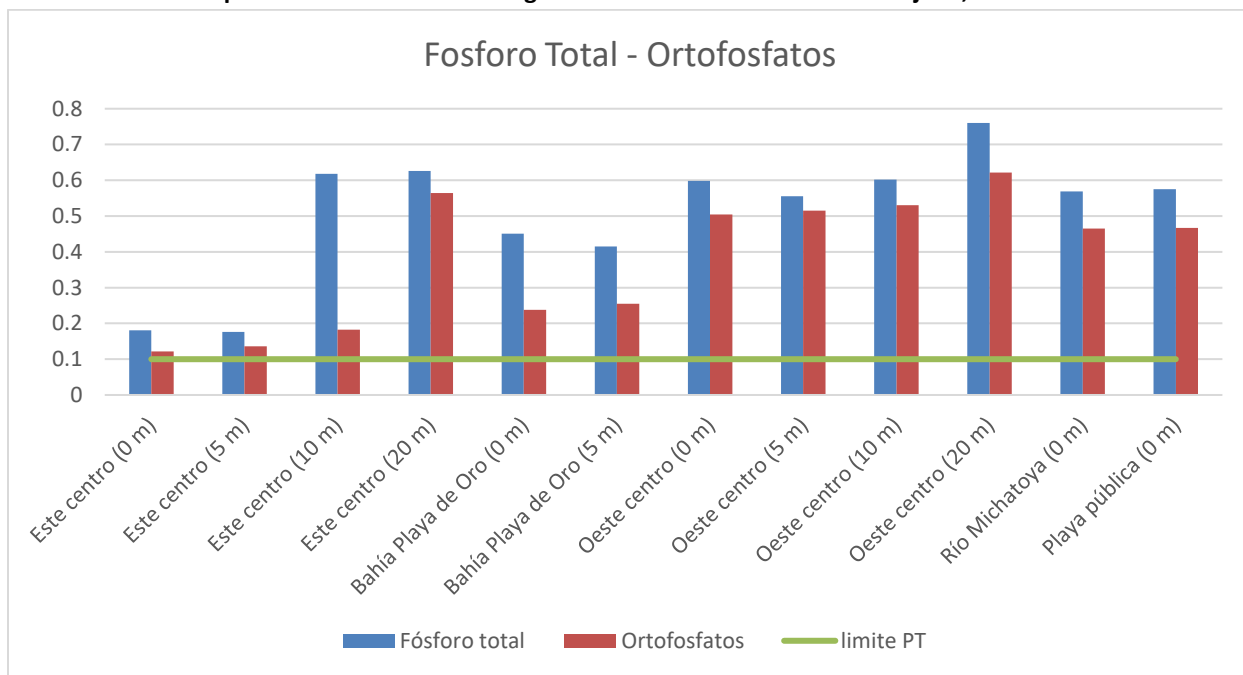
Gráfica 15: Valores de fósforo total (PT), ortofosfatos (PO4-P) y fósforo total disuelto (PTD) detectados en cinco puntos de monitoreo del lago de Amatitlán durante el mes de julio, 2024.
