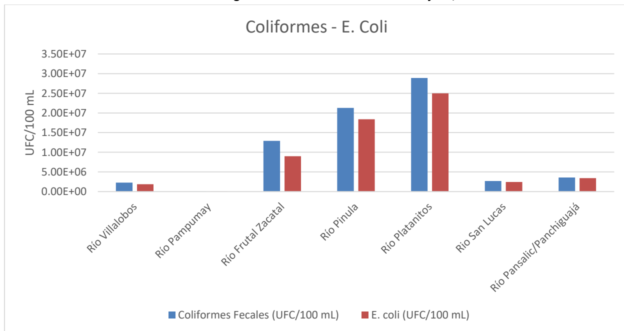
Gráfica 11: Valores de Coliformes fecales y Escherichia coli (UFC/100 ml) detectados en los ríos monitoreados en la Cuenca del Lago de Amatitlán durante el mes de julio, 2024.
