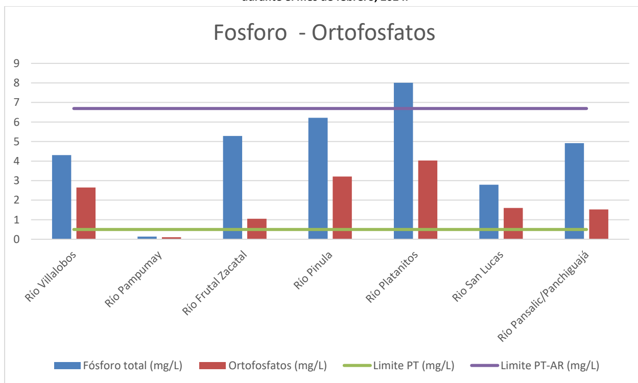
Gráfica 8: Valores de fósforo total (P) y ortofosfatos (PO4-P) de los ríos monitoreados en la Cuenca del Lago de Amatitlán durante el mes de febrero, 2024.
