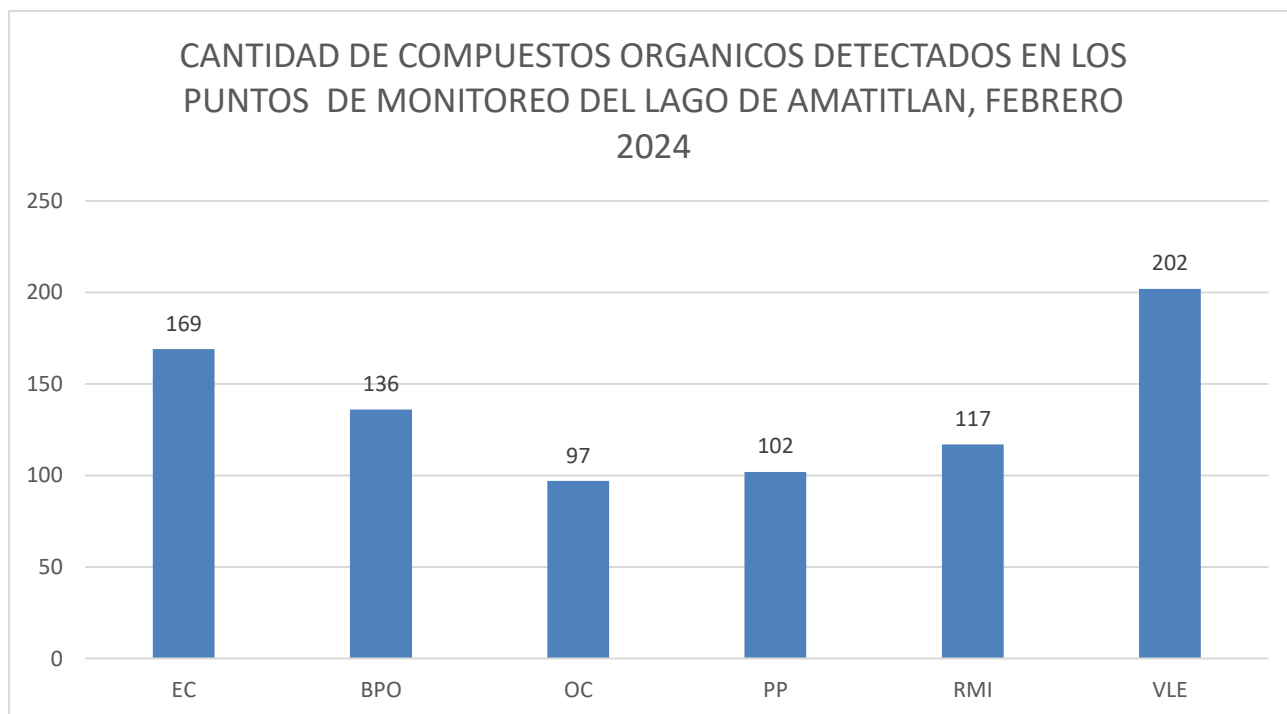
Gráfica 18: Cantidad de Sustancias Orgánicas detectadas en seis puntos de monitoreo del lago de Amatitlán durante el mes de febrero, 2024.
