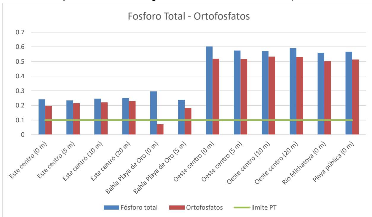
Gráfica 15: Valores de fósforo total (PT), ortofosfatos (PO4-P) y fósforo total disuelto (PTD) detectados en cinco puntos de monitoreo del lago de Amatitlán durante el mes de febrero, 2024.
