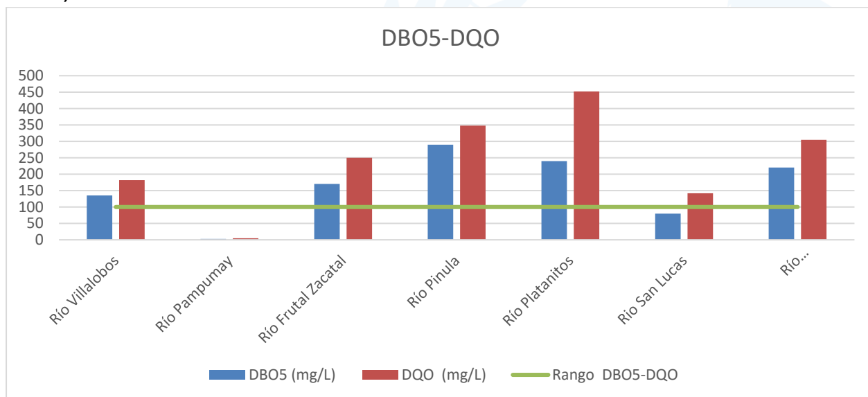
Gráfica 9: Valores de DBO 5 y DQO de los ríos muestreados de la Cuenca del lago de Amatitlán durante el mes de febrero, 2024.
