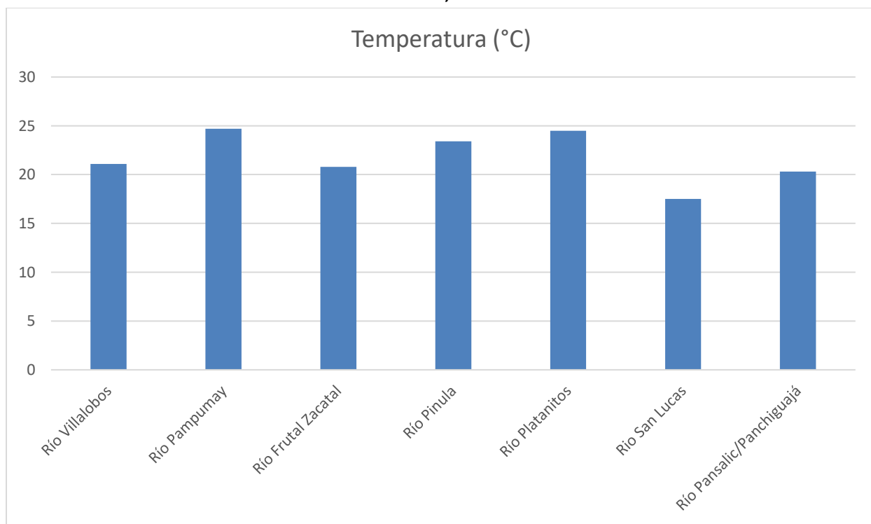
Gráfica 2: Temperatura (°C) de los ríos monitoreados en la Cuenca del Lago de Amatitlán durante el mes de febrero, 2024.
