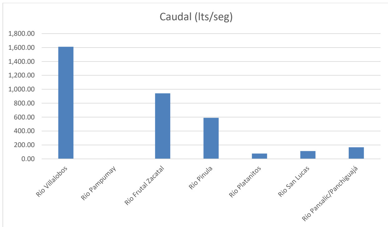
Gráfica 5: Caudal (lt/s) de los ríos monitoreados en la Cuenca del Lago de Amatitlán durante el mes de febrero, 2024.
