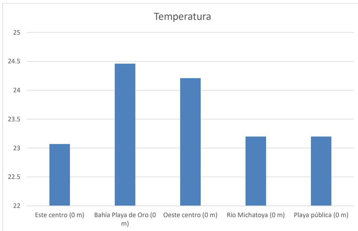
Gráfica 14: Perfil de temperatura (°C) en los puntos de monitoreo que tienen profundidad en el lago de Amatitlán (Este y Oeste Centro), durante el mes de febrero, 2024.
