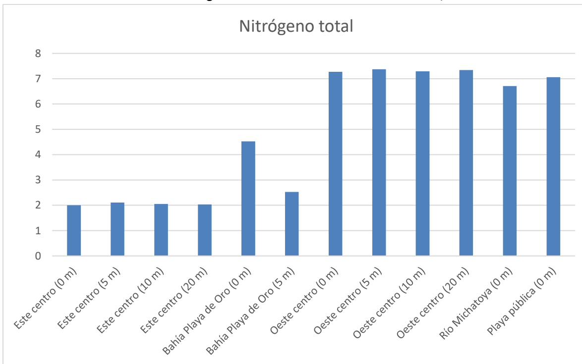
Gráfica 16: Valores de nitrógeno total (NT) y nitrógeno total disuelto (NTD) detectados en cinco puntos de monitoreo del lago de Amatitlán durante el mes de febrero, 2024.
