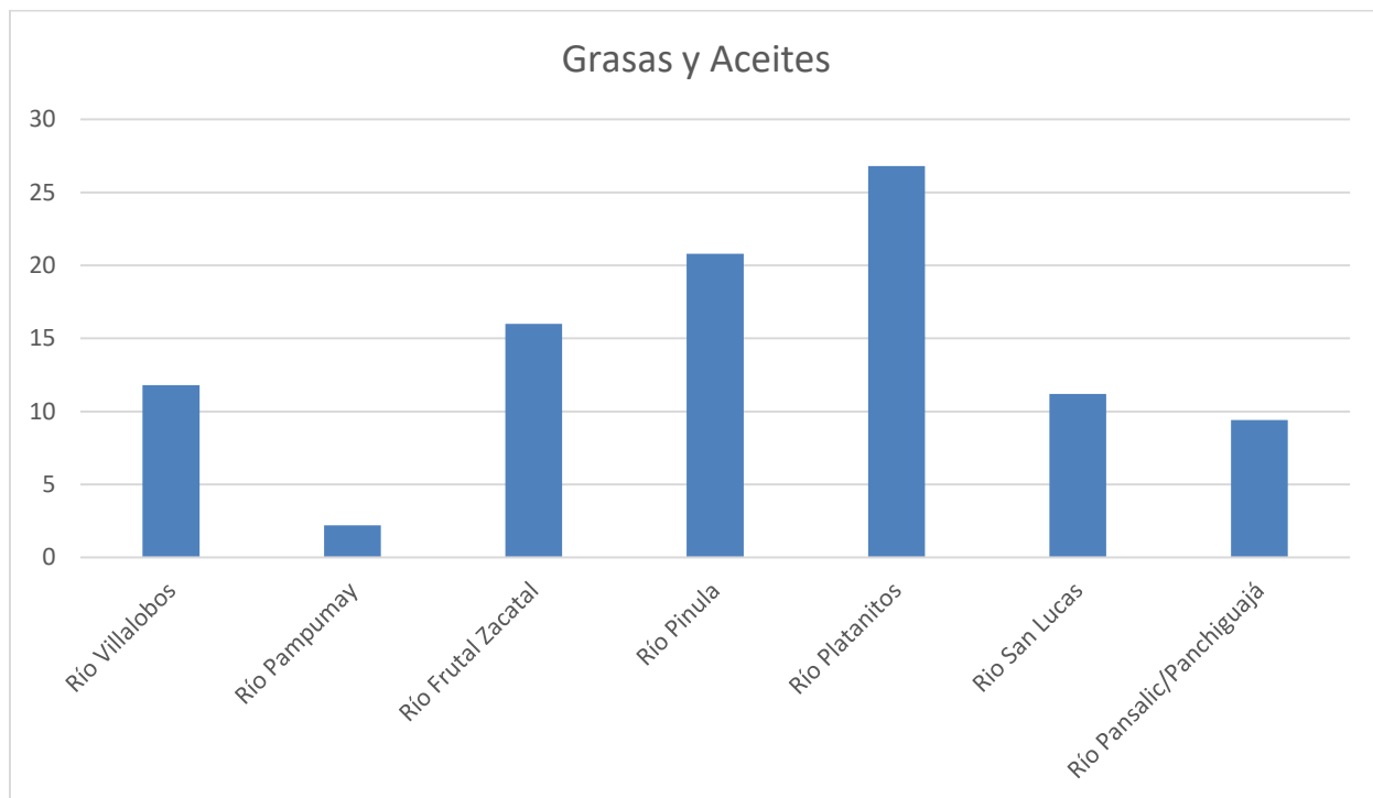
Gráfica 10: Valores de grasas y aceites (mg/L) en los ríos monitoreados de la cuenca del lago de Amatitlán durante el mes de febrero, 2024.
