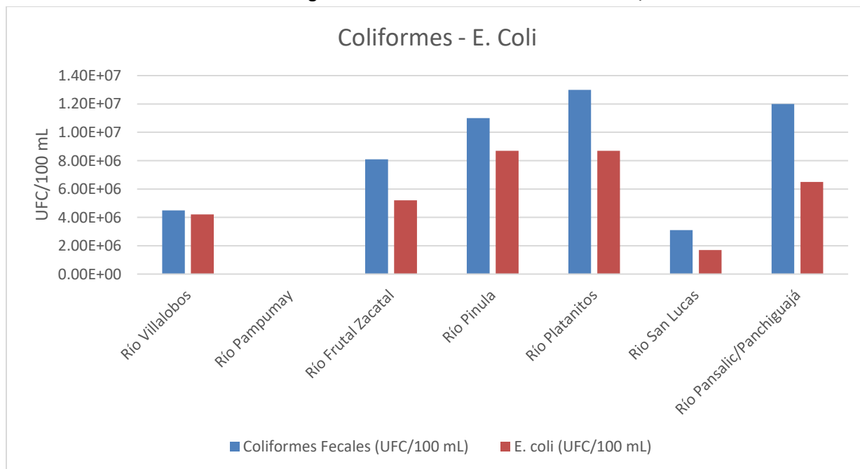
Gráfica 11: Valores de Coliformes fecales y Escherichia coli (UFC/100 ml) detectados en los ríos monitoreados en la Cuenca del Lago de Amatitlán durante el mes de febrero, 2024.
