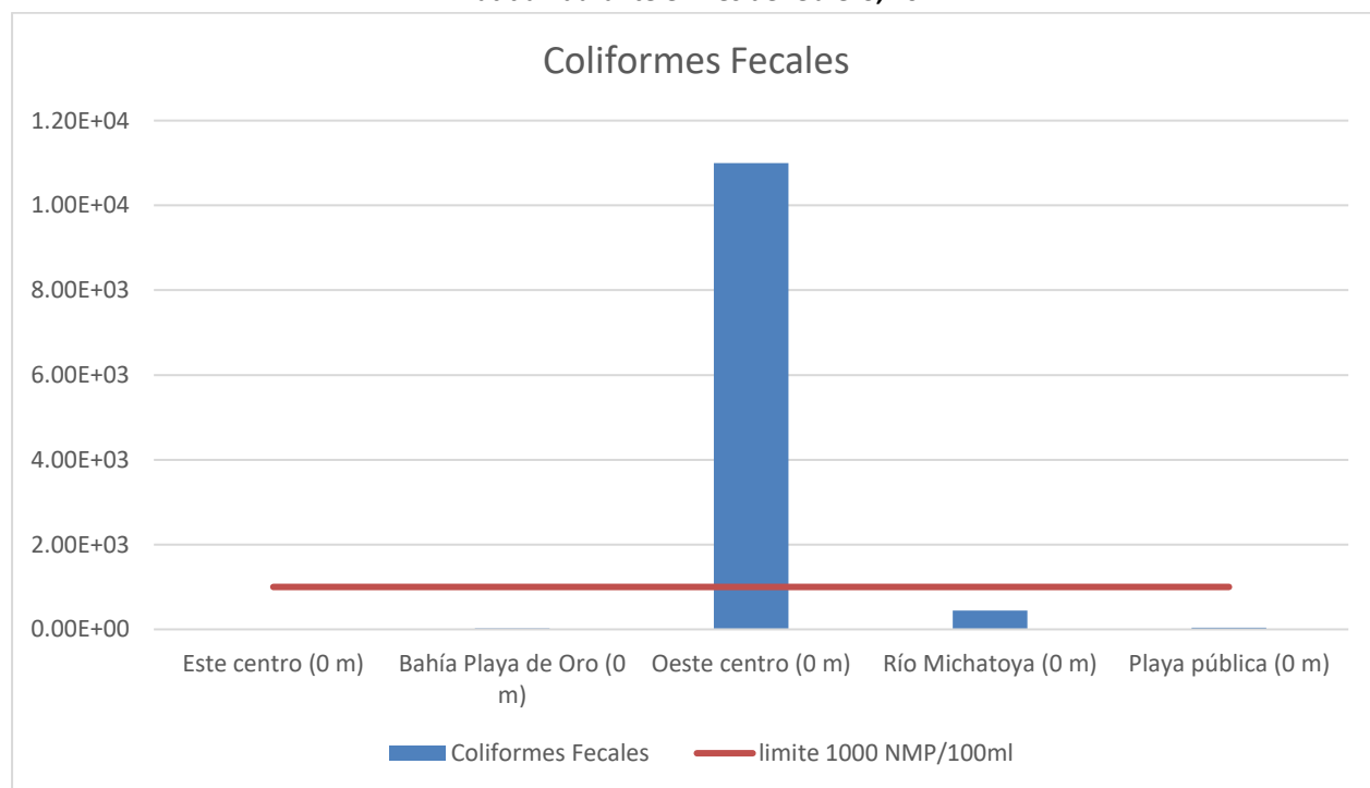
Gráfica 20: Valores de coliformes fecales (UFC/100 ml) registrados en cinco puntos de monitoreo del lago de Amatitlán durante el mes de febrero, 2024.
