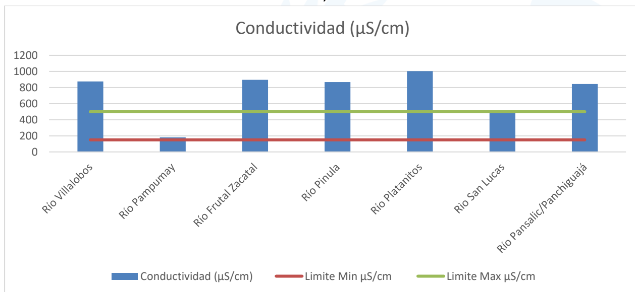
Gráfica 3: Conductividad ( \mu\text{S}/\text{cm} ) de los ríos monitoreados en la Cuenca del Lago de Amatitlán durante el mes de febrero, 2024.
