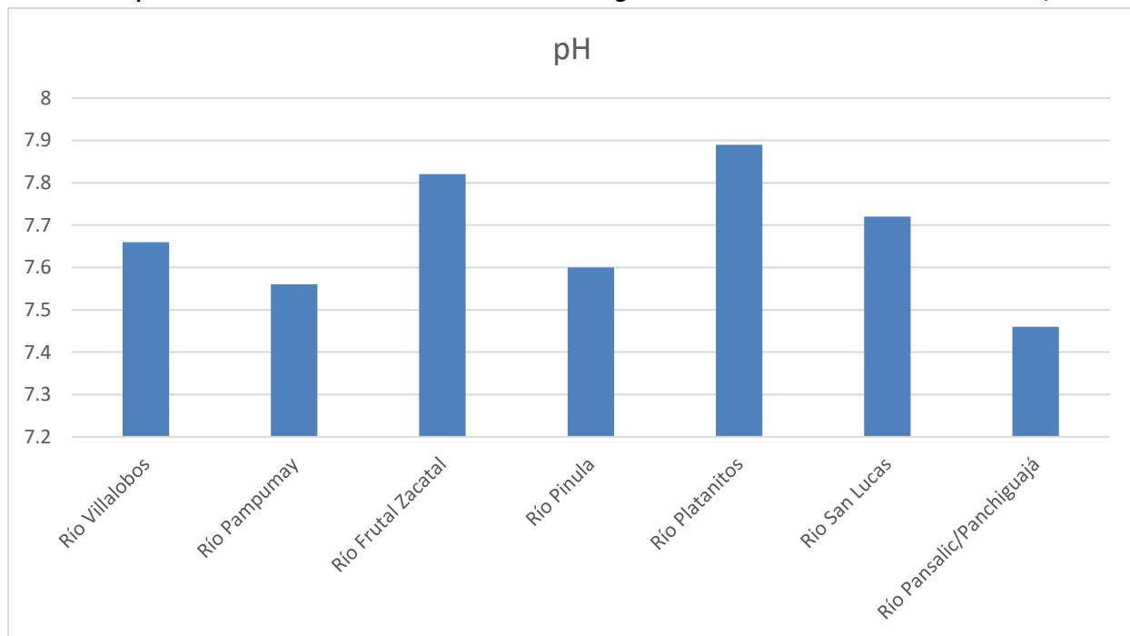
Gráfica 1: pH de los ríos monitoreados en la Cuenca del Lago de Amatitlán durante el mes de febrero, 2024.
