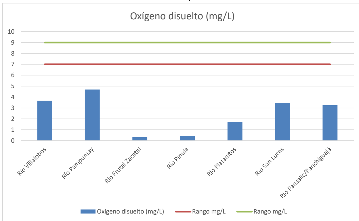
Gráfica 4: Oxígeno disuelto (mg/L) de los ríos monitoreados en la Cuenca del Lago de Amatitlán durante el mes de febrero, 2024.
