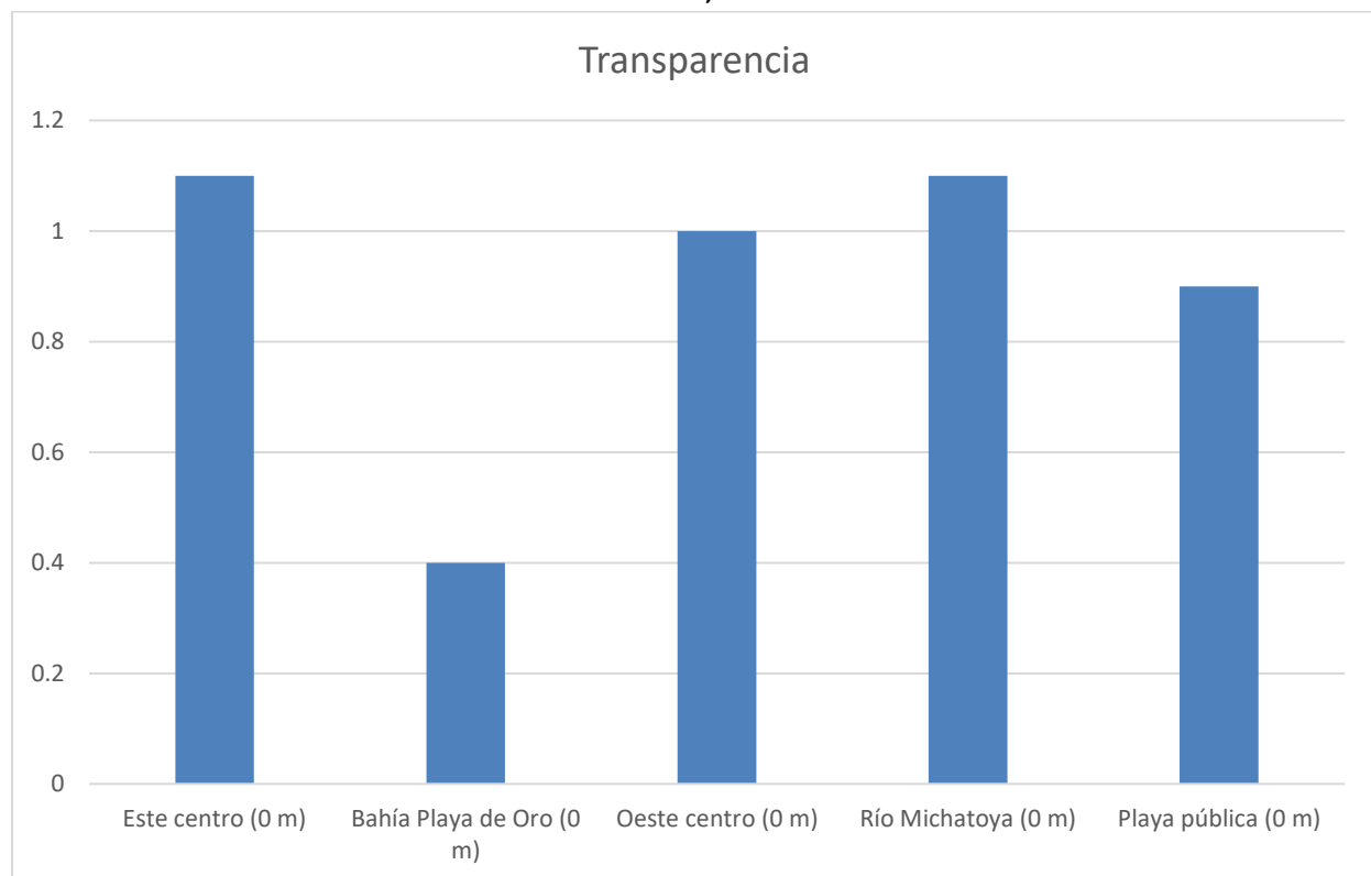
Gráfica 12: Transparencia (m) registrada en cinco puntos de monitoreo del lago de Amatitlán durante el mes de febrero, 2024
