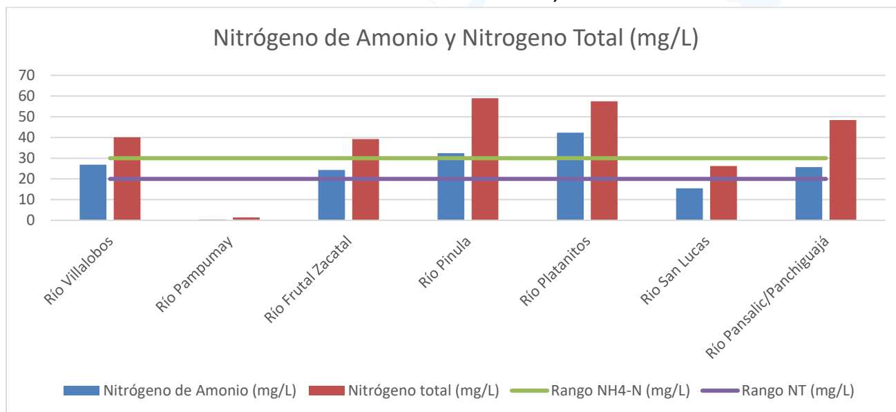
Gráfica 6: Valores de nitrógeno total (N) y amonio (NH 3 -N) de los ríos monitoreados en la Cuenca del Lago de Amatitlán durante el mes de febrero, 2024.
