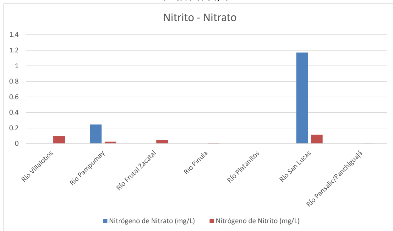
Gráfica 7: Valores de nitratos (NO 3 -N) y nitritos (NO 2 -N) de los ríos monitoreados en la Cuenca del Lago de Amatitlán durante el mes de febrero, 2024.
