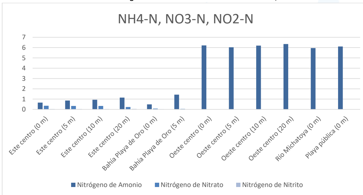
Gráfica 17: Valores de amonio (NH 4 -N), nitratos (NO 3 -N) y nitritos (NO 2 -N) detectados en cinco puntos de monitoreo del lago de Amatitlán durante el mes de febrero, 2024.
