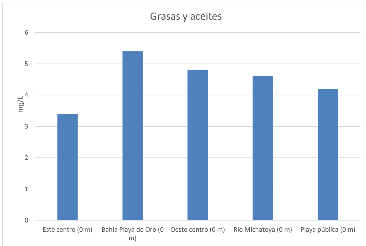
Gráfica 19: Valores de grasas y aceites (mg/L) registrados en cinco puntos de monitoreo del lago de Amatitlán durante el mes de febrero, 2024.
