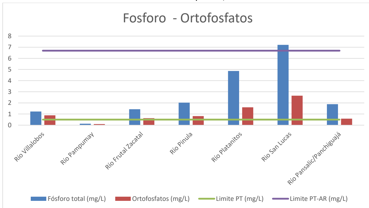
Gráfica 8: Valores de fósforo total (P) y ortofosfatos (PO4-P) de los ríos monitoreados en la Cuenca del Lago de Amatitlán durante el mes de septiembre, 2024.
