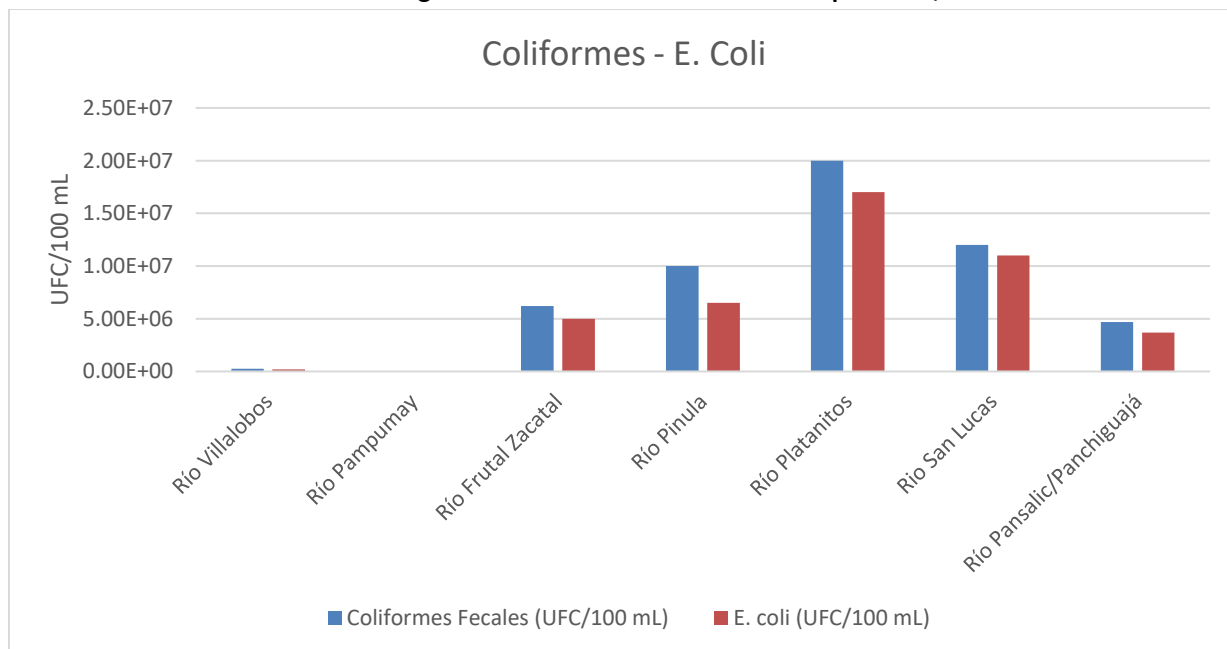
Gráfica 11: Valores de Coliformes fecales y Escherichia coli (UFC/100 ml) detectados en los ríos monitoreados en la Cuenca del Lago de Amatitlán durante el mes de septiembre, 2024.
