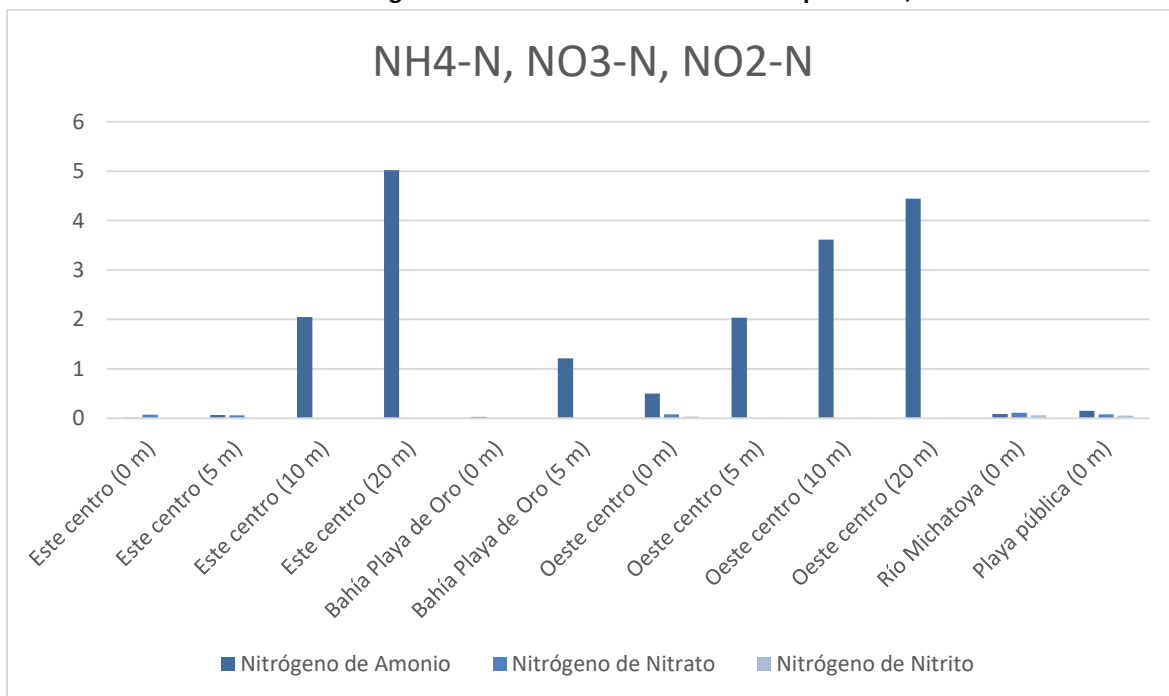
Gráfica 17: Valores de amonio (NH 4 -N), nitratos (NO 3 -N) y nitritos (NO 2 -N) detectados en cinco puntos de monitoreo del lago de Amatitlán durante el mes de septiembre, 2024.
