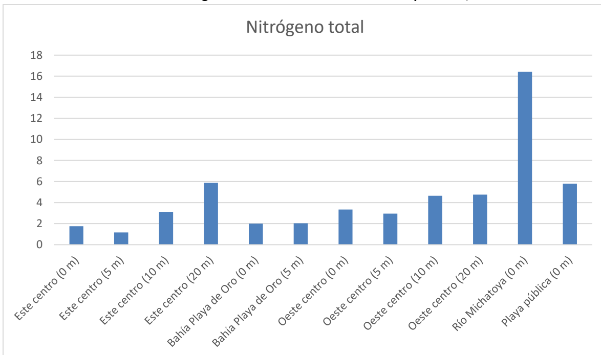
Gráfica 16: Valores de nitrógeno total (NT) y nitrógeno total disuelto (NTD) detectados en cinco puntos de monitoreo del lago de Amatitlán durante el mes de septiembre, 2024.
