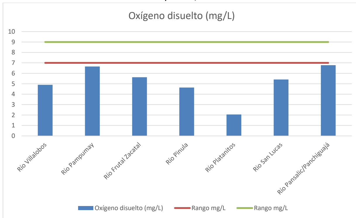
Gráfica 4: Oxígeno disuelto (mg/L) de los ríos monitoreados en la Cuenca del Lago de Amatitlán durante el mes de septiembre, 2024.
