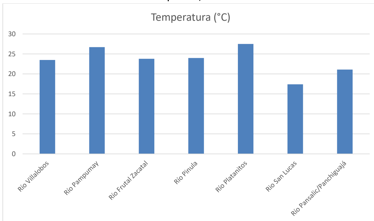
Gráfica 2: Temperatura (°C) de los ríos monitoreados en la Cuenca del Lago de Amatitlán durante el mes de septiembre, 2024.
