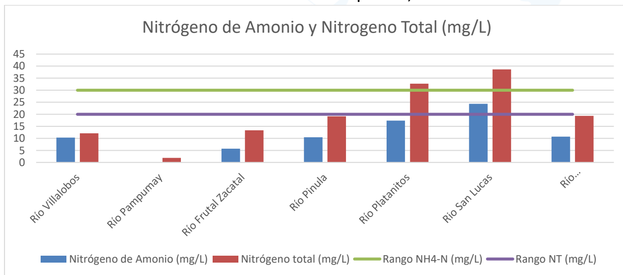
Gráfica 6: Valores de nitrógeno total (N) y amonio (NH 3 -N) de los ríos monitoreados en la Cuenca del Lago de Amatitlán durante el mes de septiembre, 2024.
