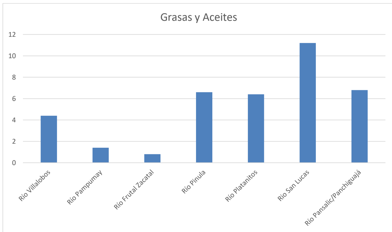
Gráfica 10: Valores de grasas y aceites (mg/L) en los ríos monitoreados de la cuenca del lago de Amatitlán durante el mes de septiembre, 2024.
