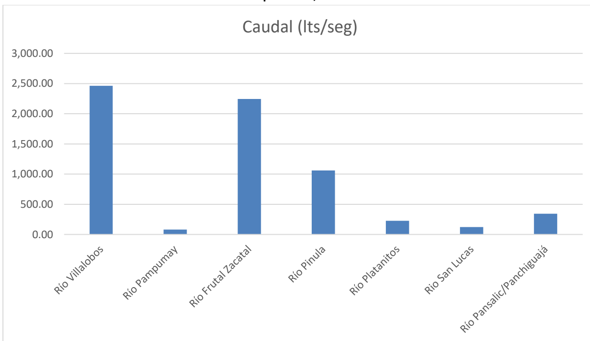
Gráfica 5: Caudal (lt/s) de los ríos monitoreados en la Cuenca del Lago de Amatitlán durante el mes de septiembre, 2024.
