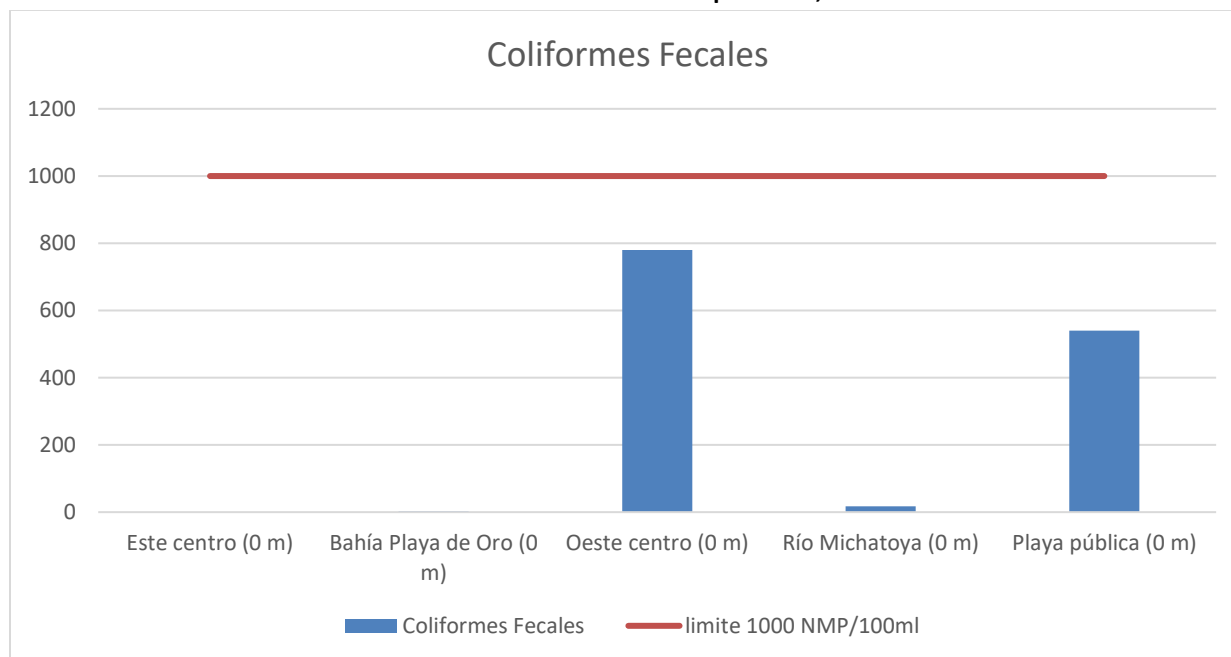
Gráfica 19: Valores de coliformes fecales (UFC/100 ml) registrados en cinco puntos de monitoreo del lago de Amatitlán durante el mes de septiembre, 2024.
