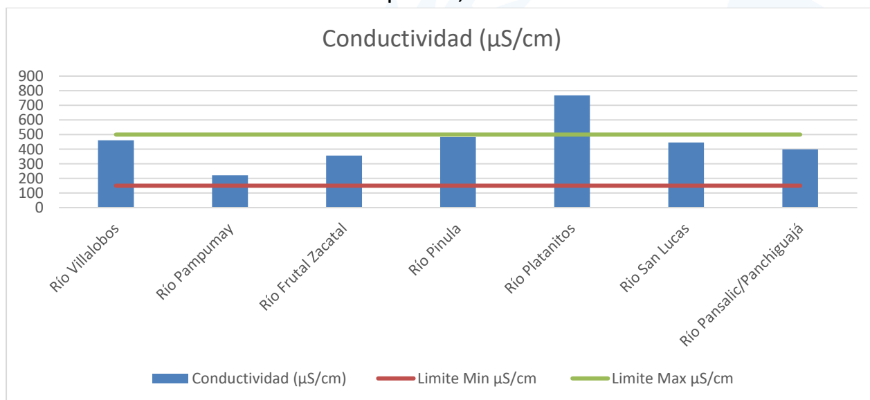
Gráfica 3: Conductividad ( \mu\text{S}/\text{cm} ) de los ríos monitoreados en la Cuenca del Lago de Amatitlán durante el mes de septiembre, 2024.
