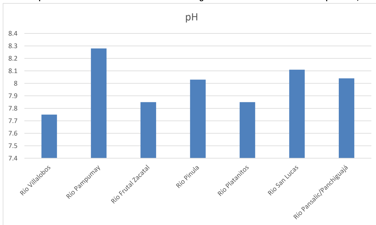
Gráfica 1: pH de los ríos monitoreados en la Cuenca del Lago de Amatitlán durante el mes de septiembre, 2024.
