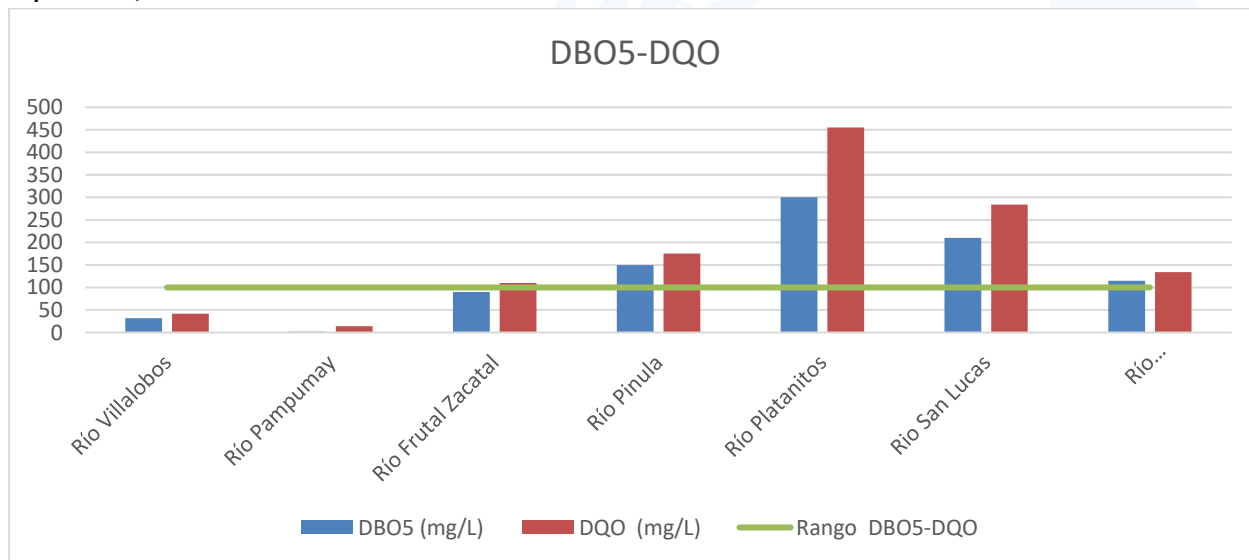
Gráfica 9: Valores de DBO 5 y DQO de los ríos muestreados de la Cuenca del lago de Amatitlán durante el mes de septiembre, 2024.
