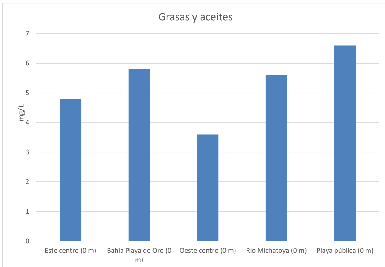
Gráfica 18: Valores de grasas y aceites (mg/L) registrados en cinco puntos de monitoreo del lago de Amatitlán durante el mes de septiembre, 2024.
